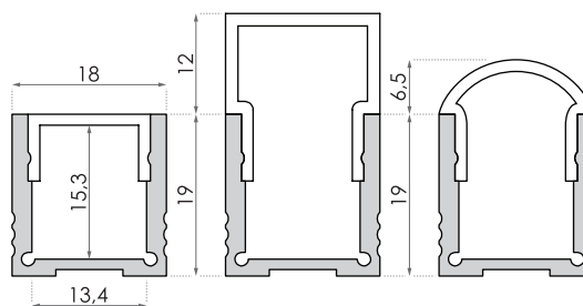
ALU profil BAR3, 18 x 19 mm *Maksimalna dolžina profila je 5 m
