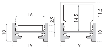
ALU profil BAR5, 19 x 10 mm Kat. št.: 5010535 *Maksimalna dolžina profila je 5 m
